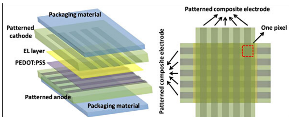
Figura 3.6: Pantalla matricial OLED para pantallas RGB
