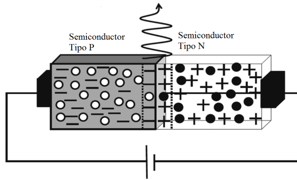
Figura 1.12: Estructura de Led inorgánico P-N bajo funcionamiento
