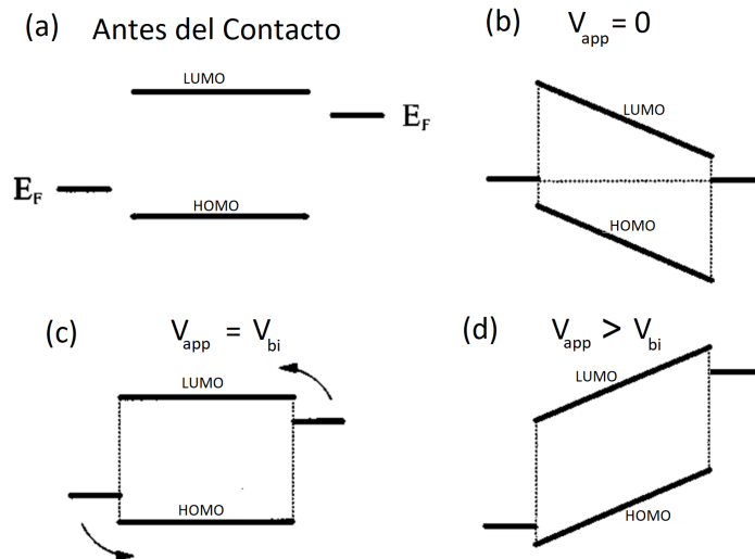
Figura 1.8: Ilustración esquemática del potencial incorporado V_{bi} en un OSC. (a) E_F representa el nivel de Fermi de los electrodos metálicos y el HOMO y LUMO del OSC separados de los contactos. (b) Al entrar en contacto los materiales, se establece una diferencia de potencial dentro del dispositivo V_{bi} que modifica el LUMO y HOMO a causa de igualación de energía de Fermi de los contactos; a mayor diferencia de energía de Fermi de los contactos, mas se distorsiona el HOMO y el LUMO. (c) Al aplicar un voltaje en polarización directa igual a la diferencia de energía de Fermi de los electrodos, permitiendo la existencia de corriente en el dispositivo. Este potencial V_{bi} debe superarse antes de que el dispositivo comience a funcionar. (d) Al aplicar un voltaje mayor que V_{bi} , no existe barrera potencial que oponga paso de electrones y huecos.
