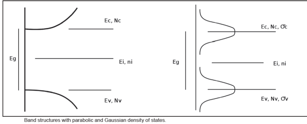
Figura 1.5: Estructuras de bandas con densidad de estados parabólica y gaussiana.
