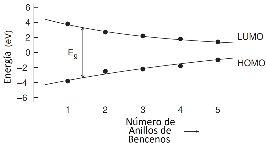
Figura 1.4: Ejemplo del GAP para bencenoides en función del tamaño molecular. Para aumentar la longitud de la conjugación, desde el benceno hasta el pentaceno, la brecha se estrecha. Este efecto es causado por un aumento de la dislocación de las cargas y se amplifica aún más cuando las moléculas están cerca unas de otras.
